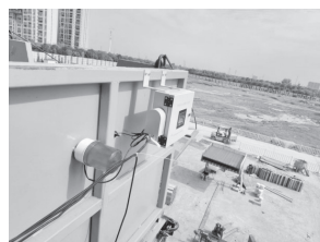
卸料平台超载报警器运用
